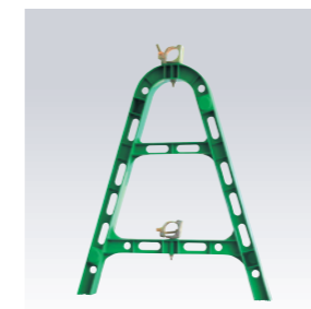
BAJG 単管バリケード(樹脂バリ) サイズ: 820mm×630mm 材質: ポリスチレン樹脂
