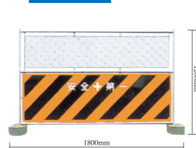
F-12A ガードフェンス LF12A
