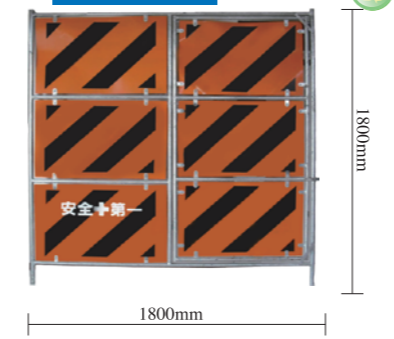
F-18TC 扉フェンス(トラ3段) LF18C
